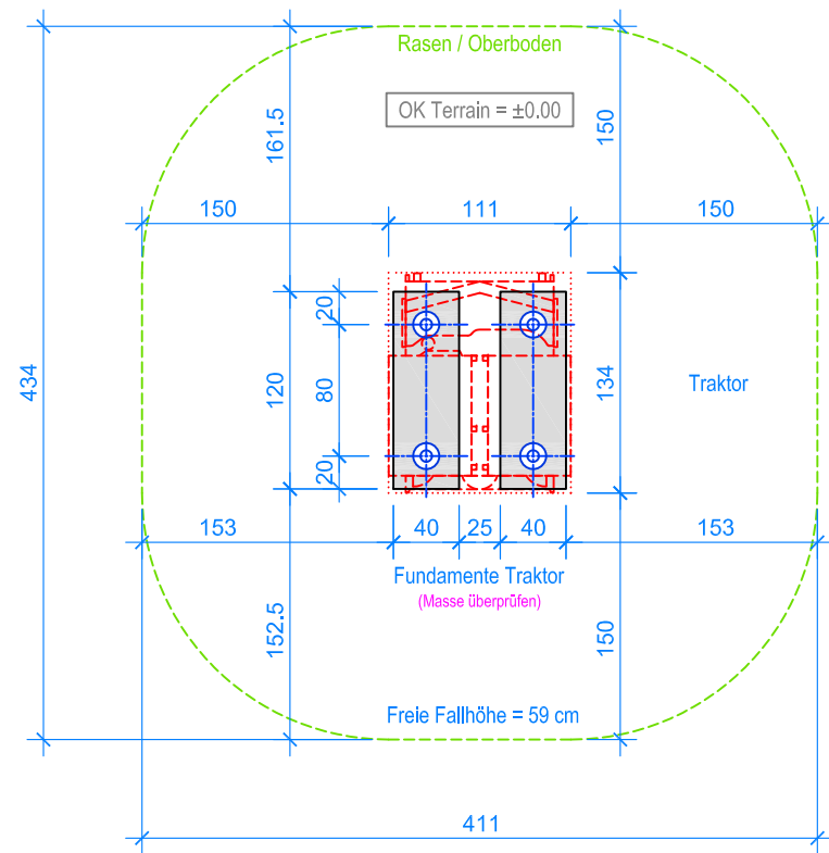
GRUNDRISS 1:50
