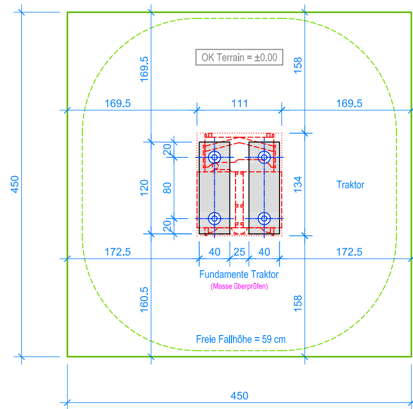
GRUNDRISS 1:50
