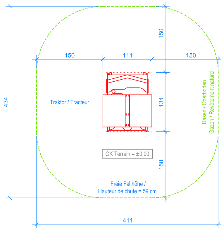
GRUNDRISS / PLAN 1:50
