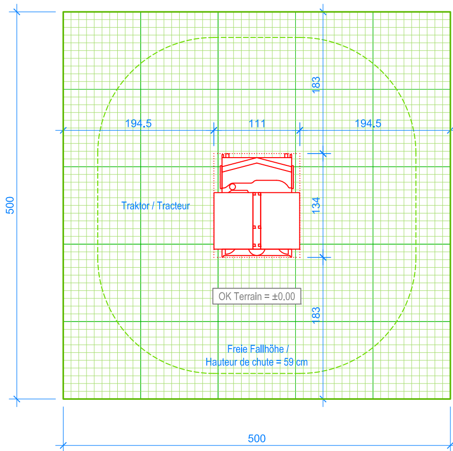
GRUNDRISS / PLAN 1:50
