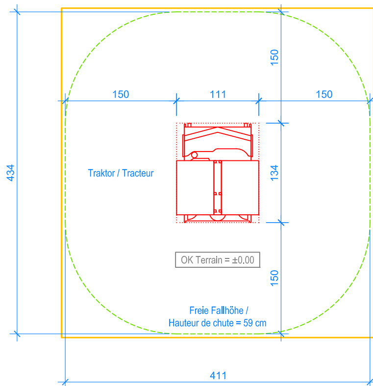
GRUNDRISS / PLAN 1:50
