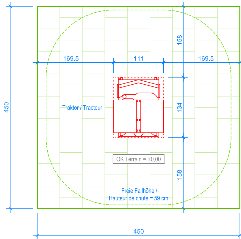
GRUNDRISS / PLAN 1:50
