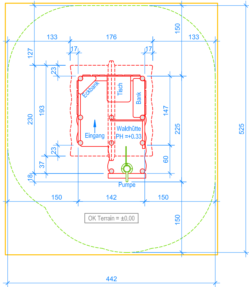
GRUNDRISS 1:50
