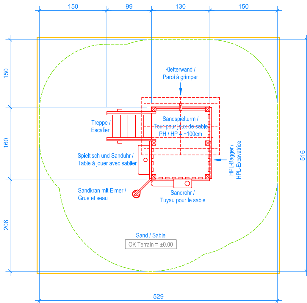
GRUNDRISS / PLAN 1:50
