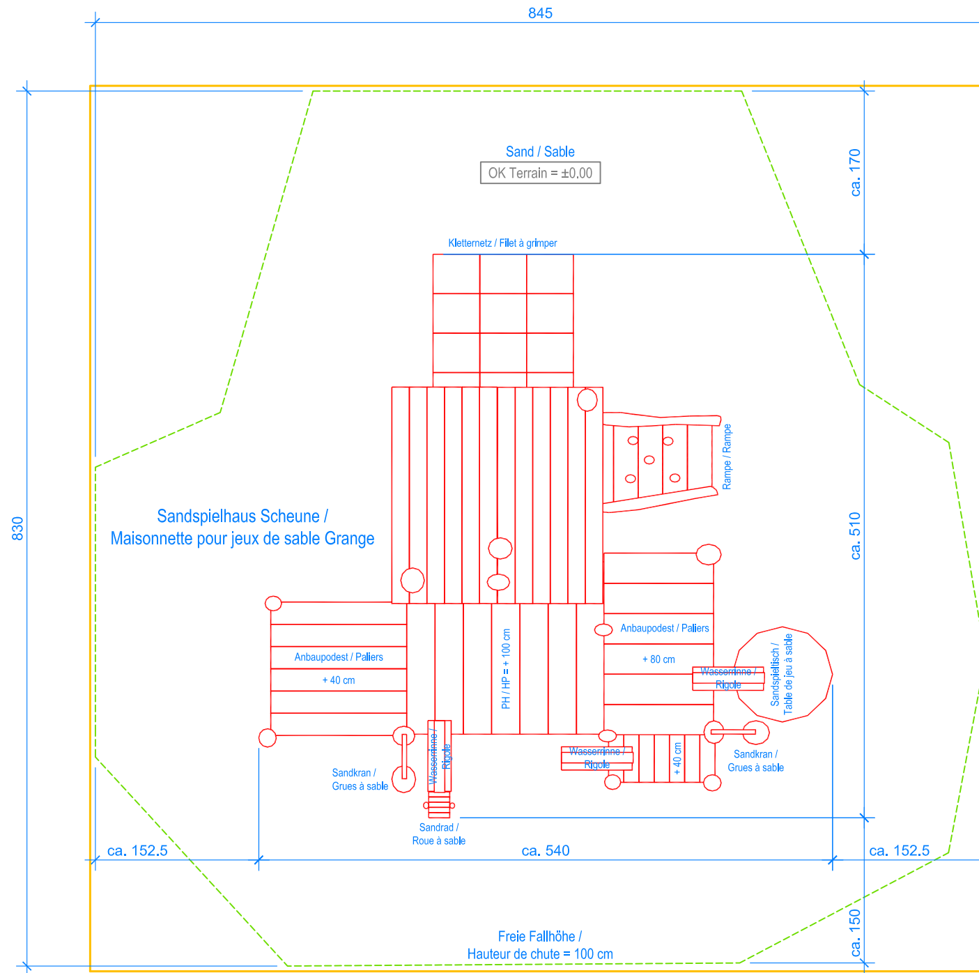
GRUNDRISS / PLAN 1:50
