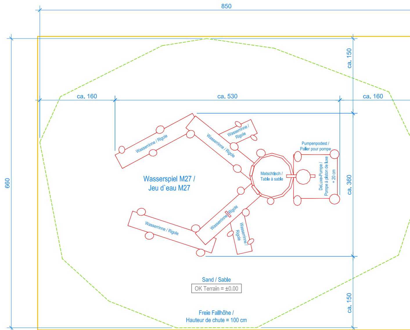
GRUNDRISS / PLAN 1:50
