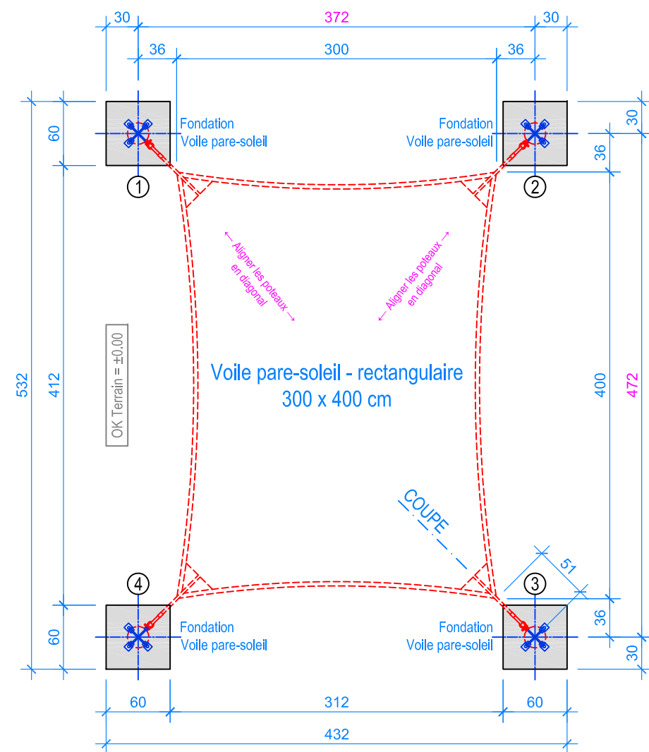
PLAN 1:50
