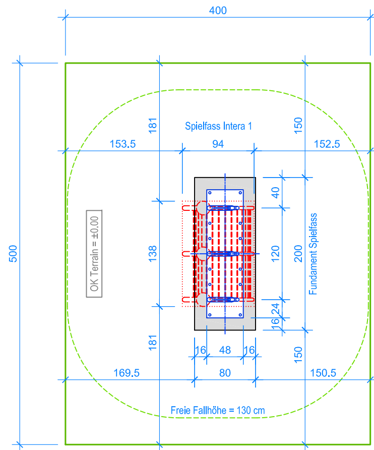
GRUNDRISS 1:50
