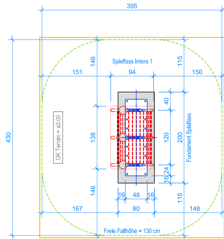
GRUNDRISS 1:50
