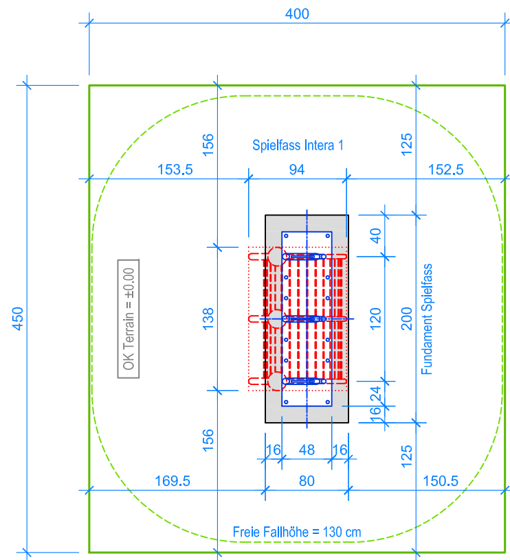
GRUNDRISS 1:50
