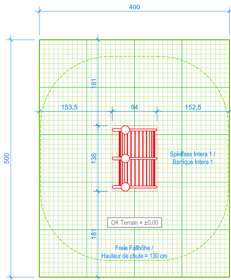
GRUNDRISS / PLAN 1:50
