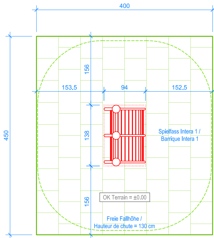
GRUNDRISS / PLAN 1:50
