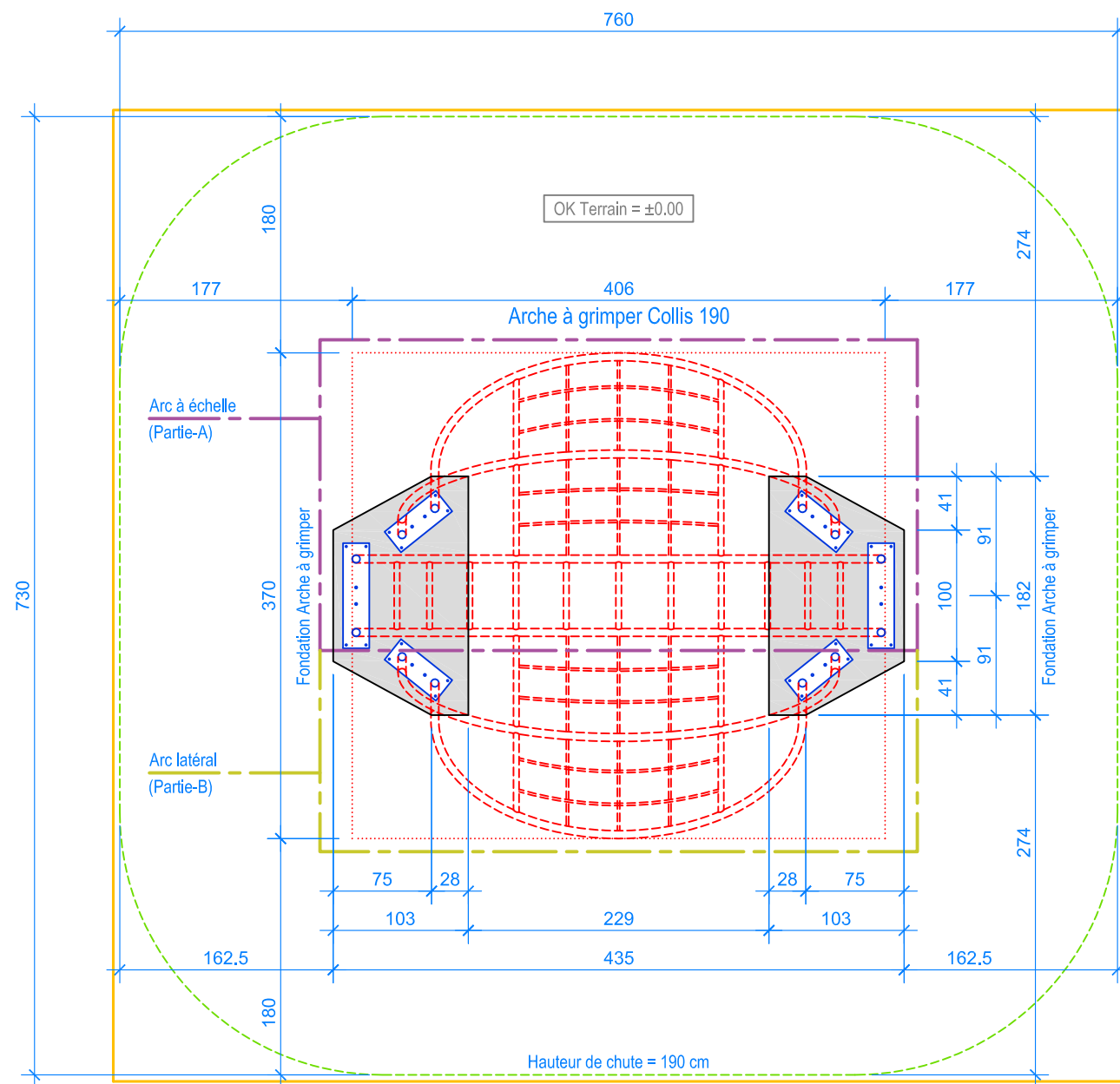
PLAN 1:50
