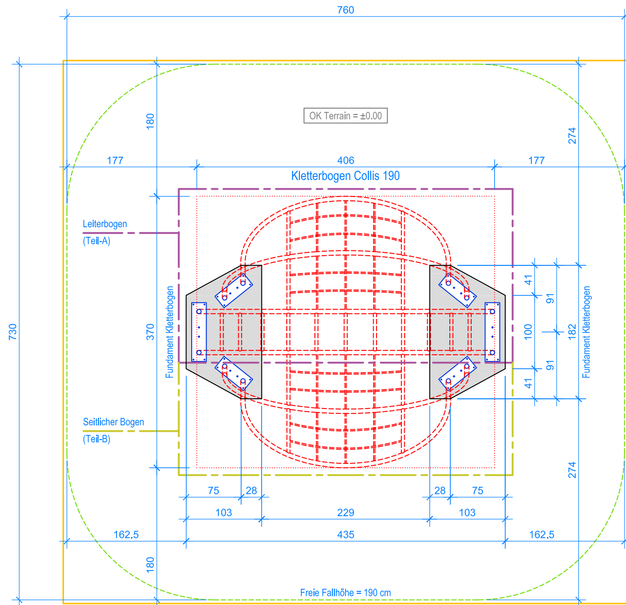
GRUNDRISS 1:50
