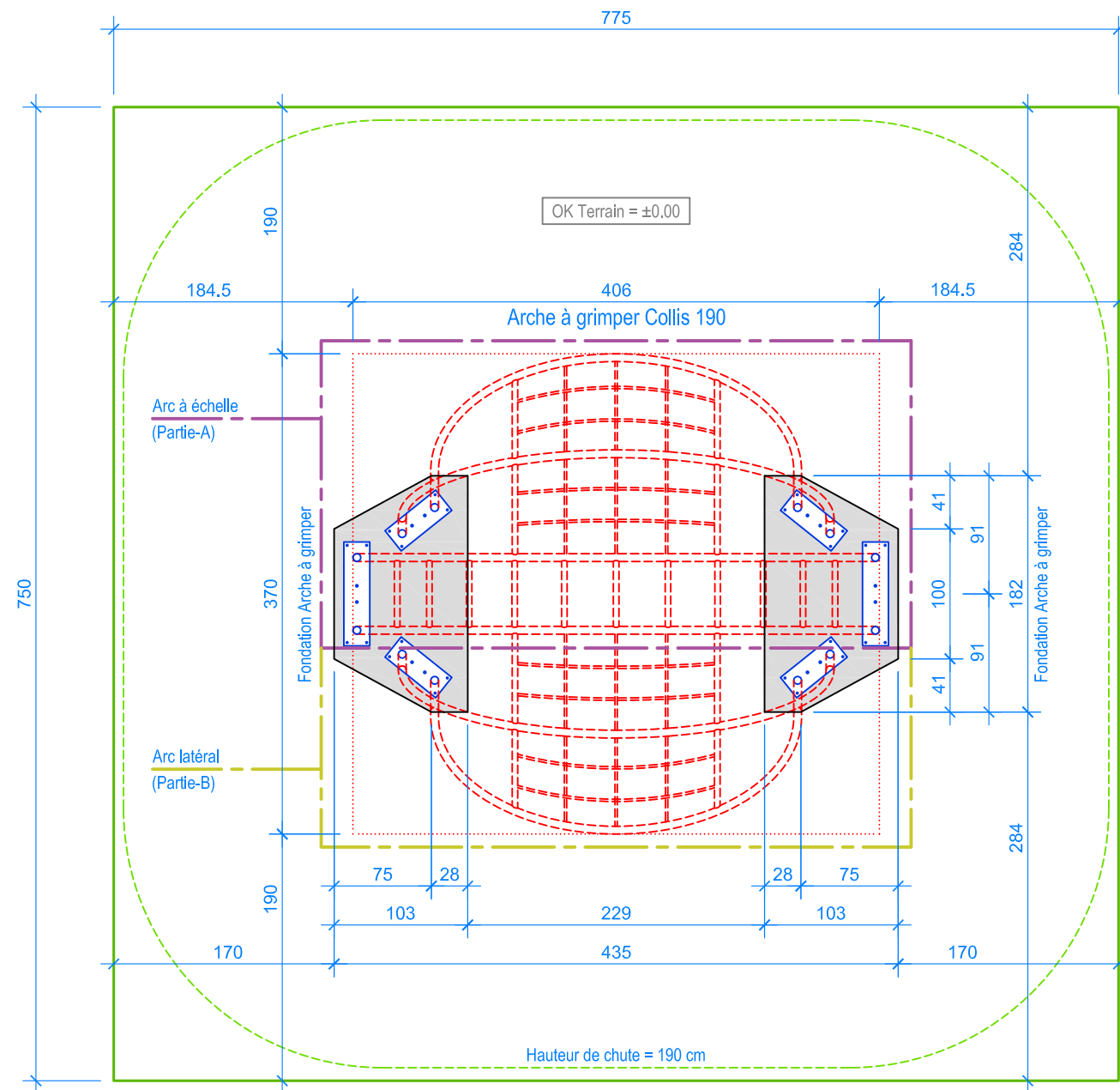
PLAN 1:50
