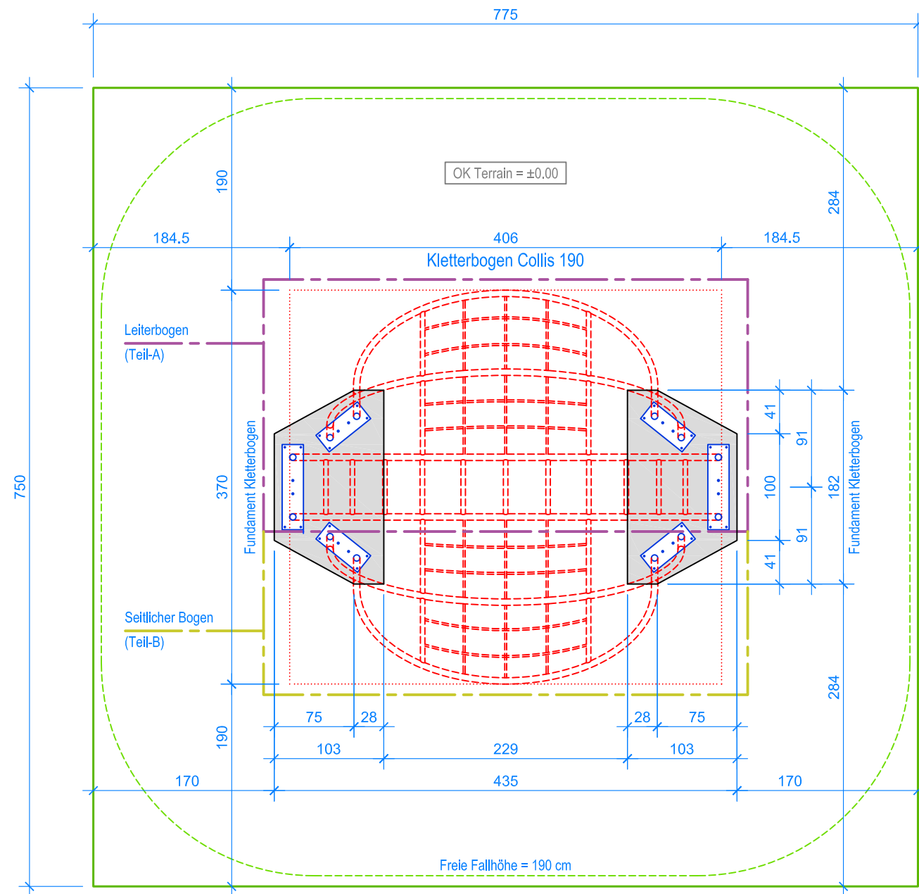
GRUNDRISS 1:50
