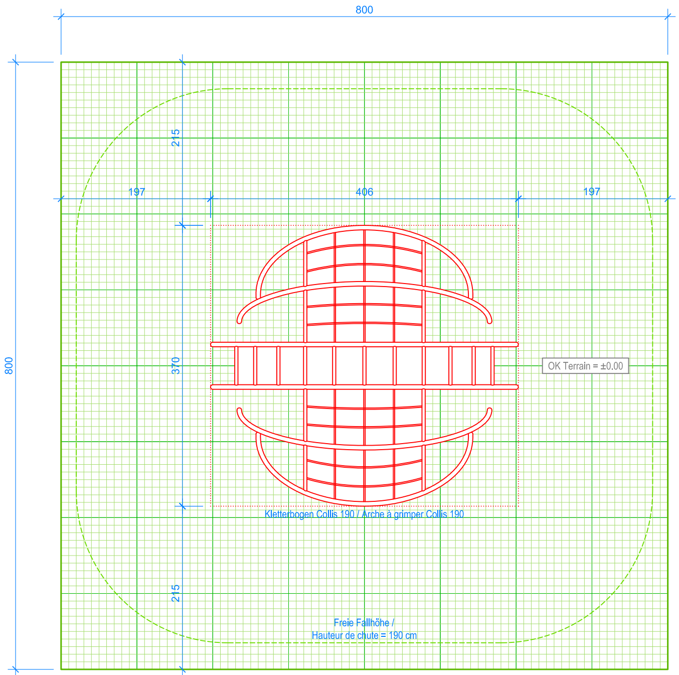
GRUNDRISS / PLAN 1:50
