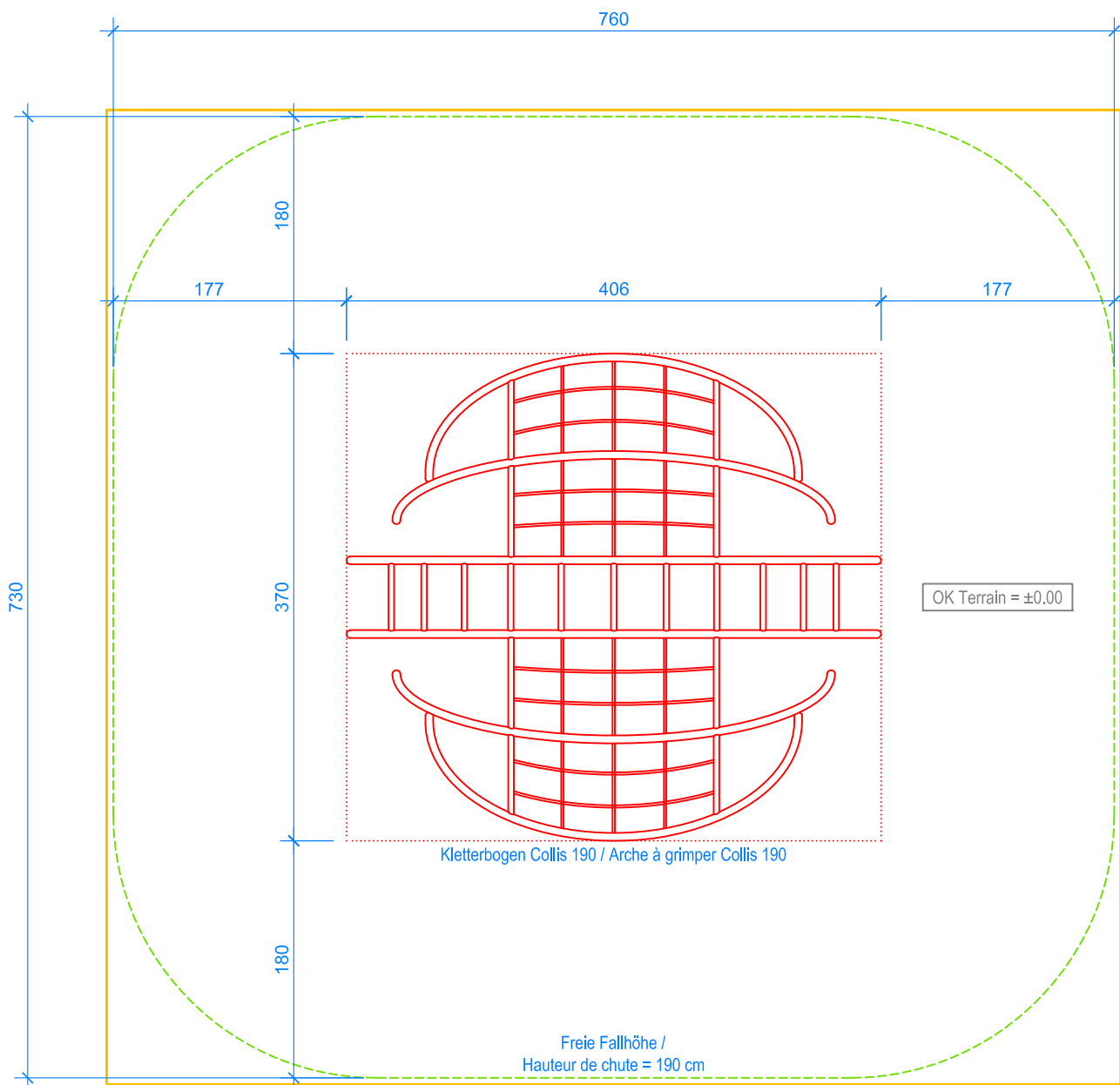
GRUNDRISS / PLAN 1:50
