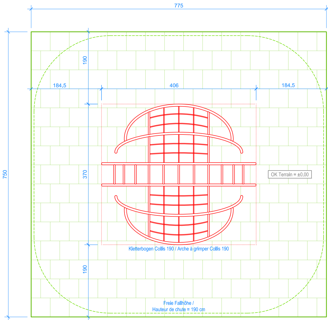
GRUNDRISS / PLAN 1:50
