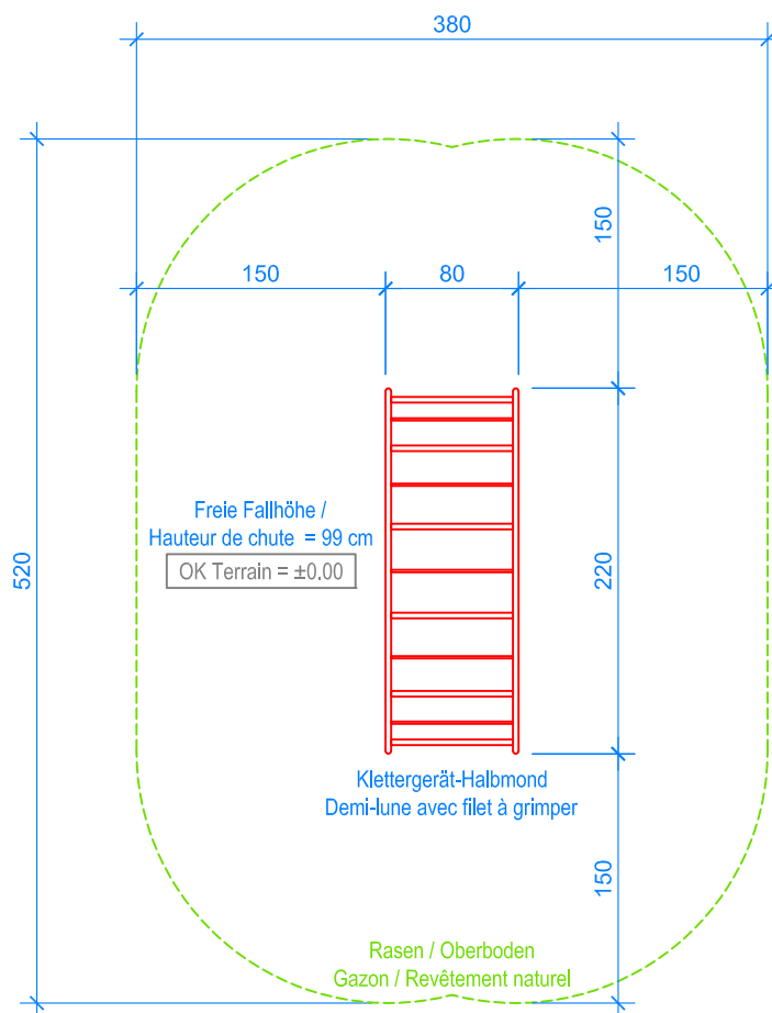
GRUNDRISS / PLAN 1:50
