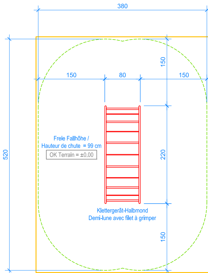
GRUNDRISS / PLAN 1:50
