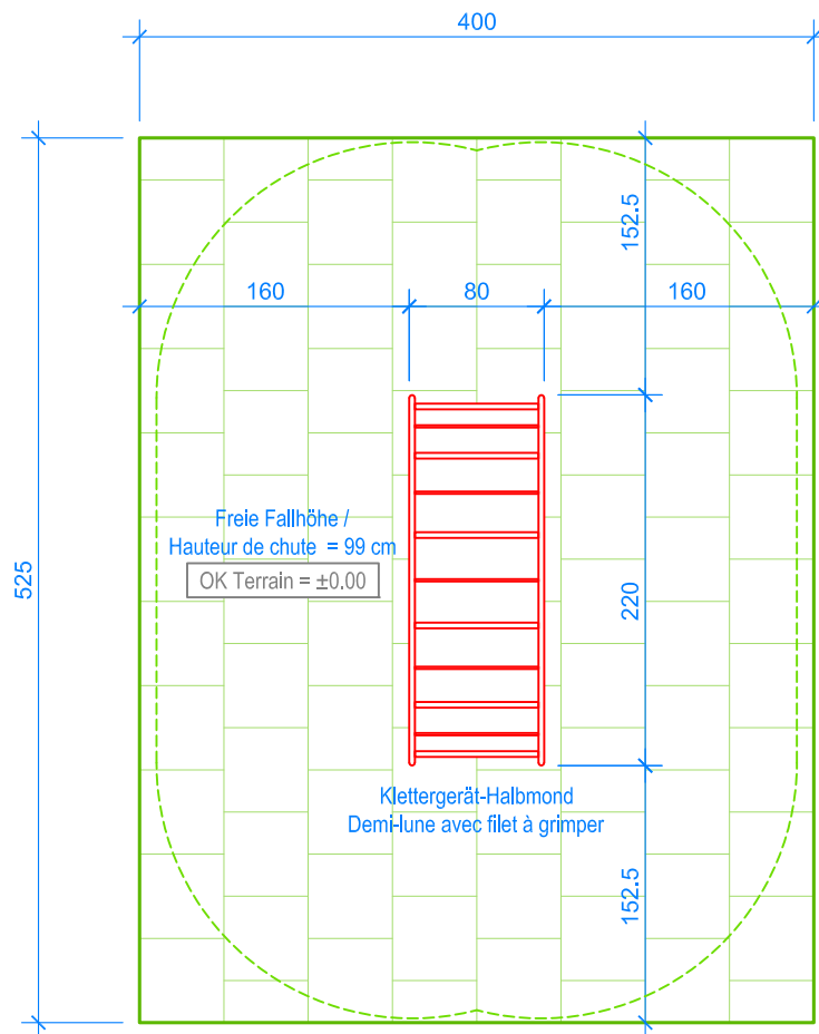
GRUNDRISS / PLAN 1:50
