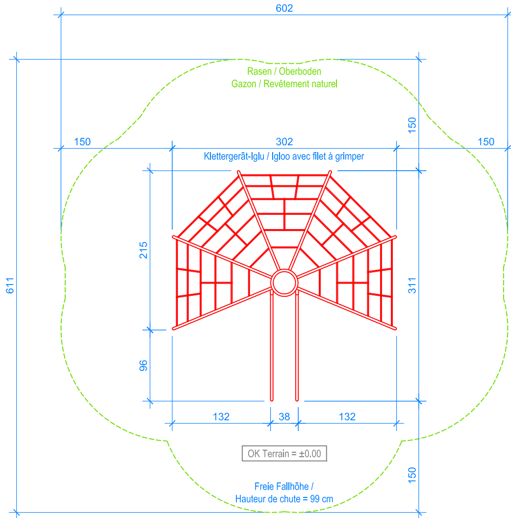
GRUNDRISS / PLAN 1:50
