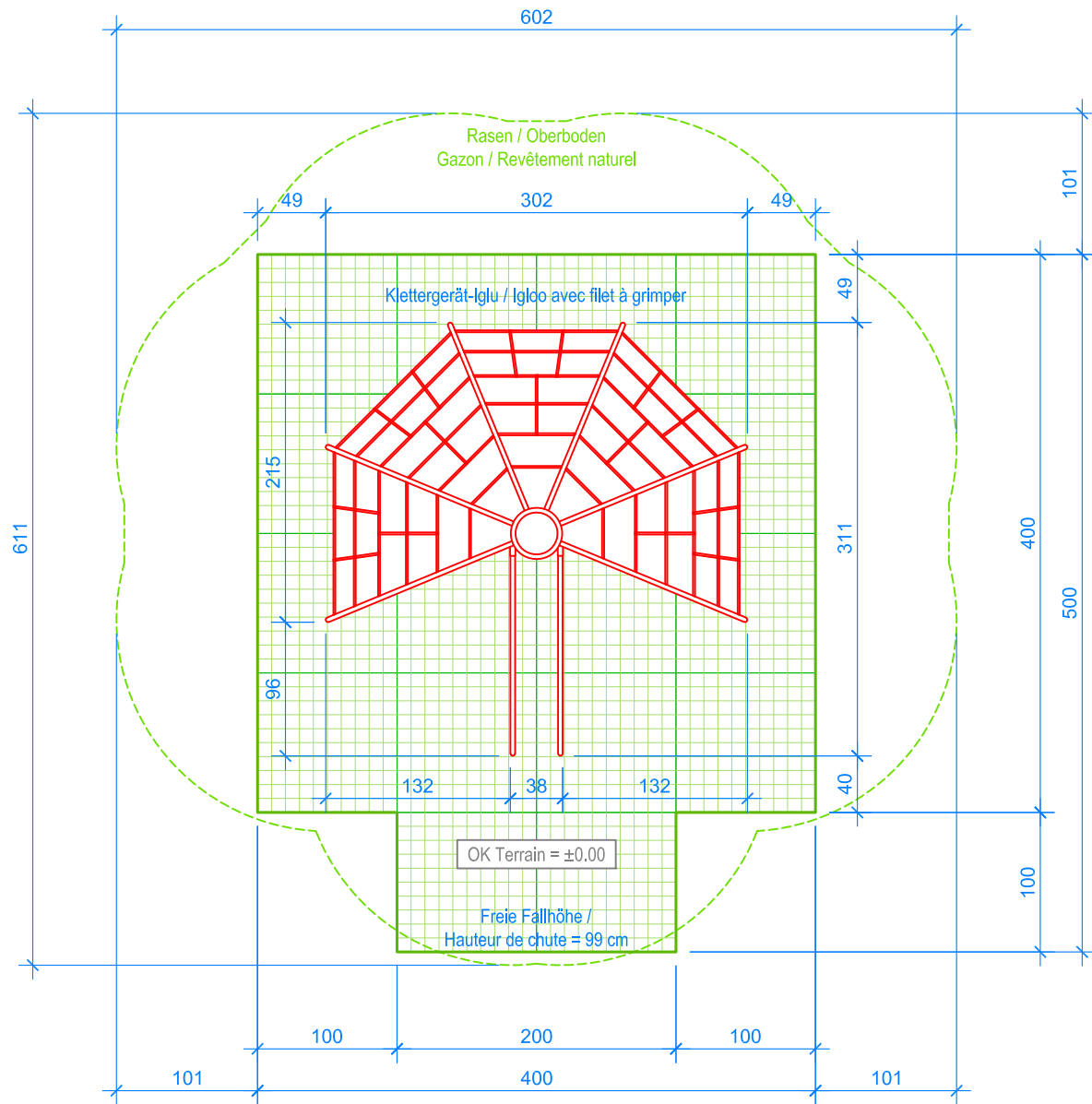
GRUNDRISS / PLAN 1:50
