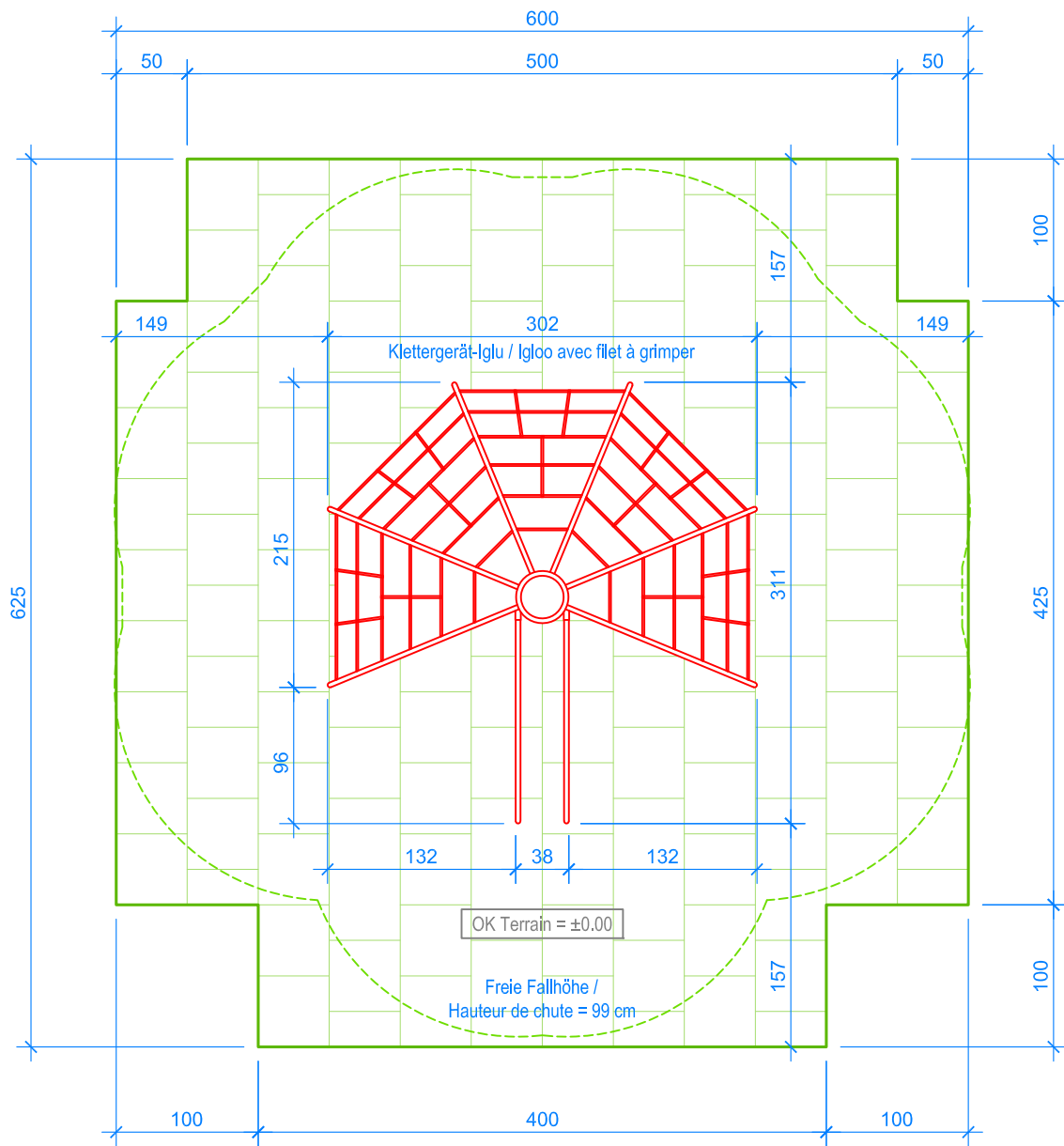
GRUNDRISS / PLAN 1:50
