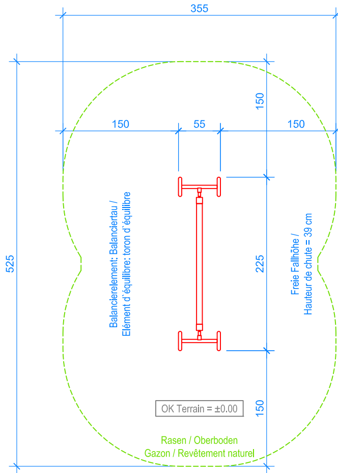
GRUNDRISS / PLAN 1:50
