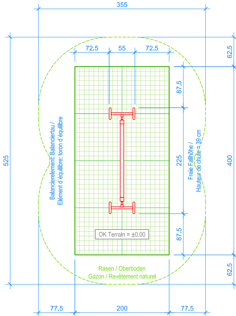
GRUNDRISS / PLAN 1:50
