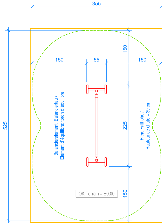
GRUNDRISS / PLAN 1:50
