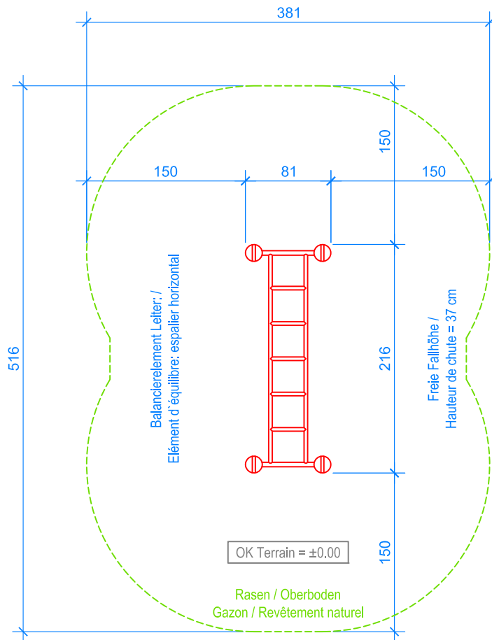
GRUNDRISS / PLAN 1:50
