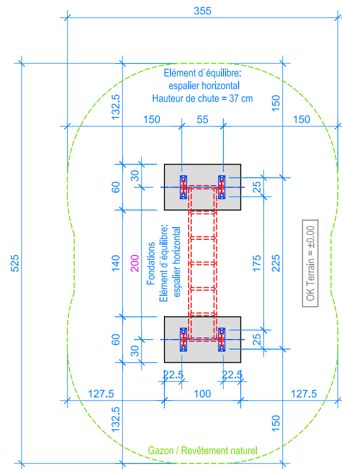
PLAN 1:50
