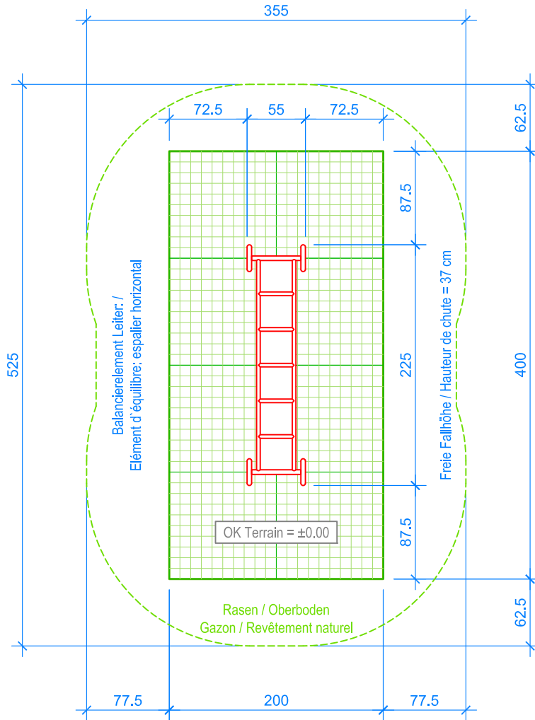
GRUNDRISS / PLAN 1:50
