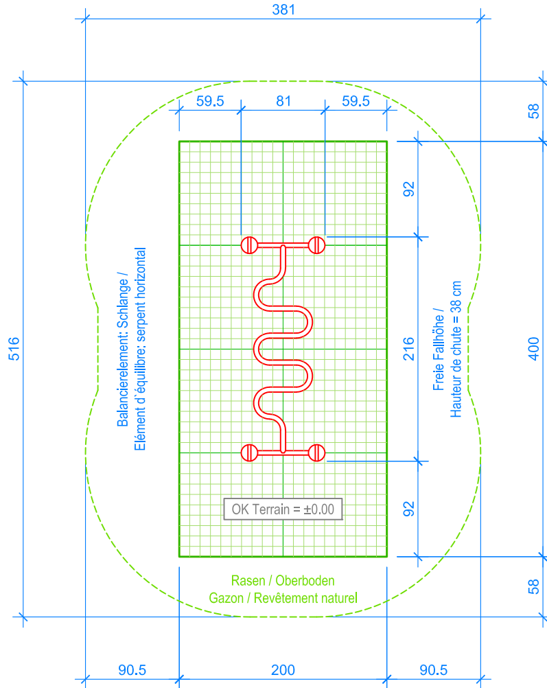
GRUNDRISS / PLAN 1:50
