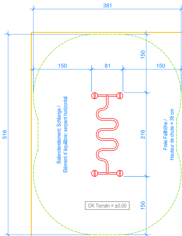
GRUNDRISS / PLAN 1:50
