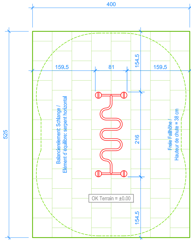
GRUNDRISS / PLAN 1:50
