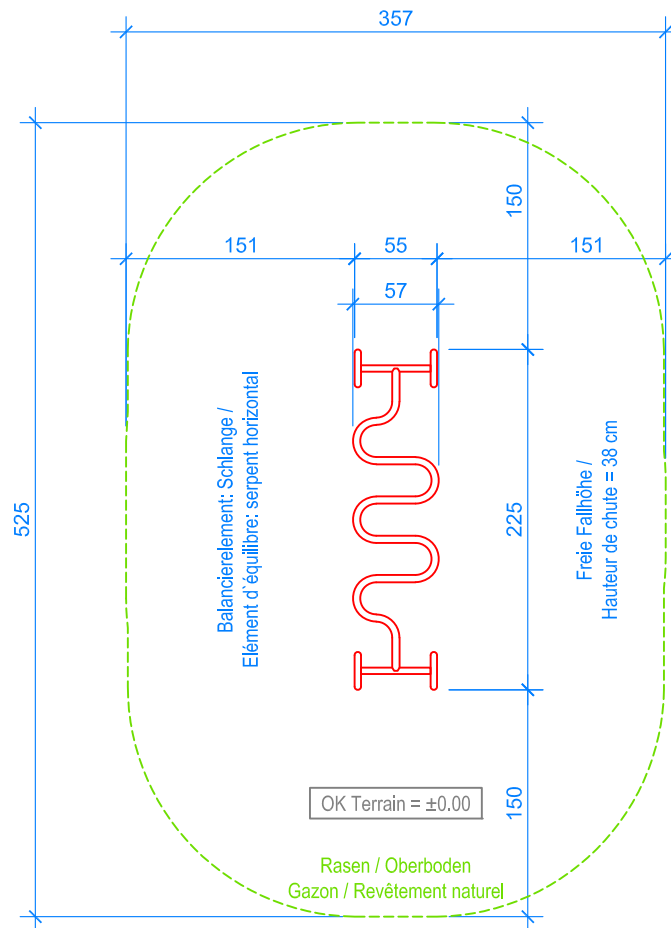
GRUNDRISS / PLAN 1:50
