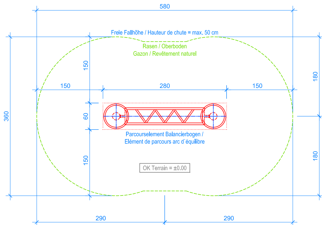
GRUNDRISS / PLAN 1:50
