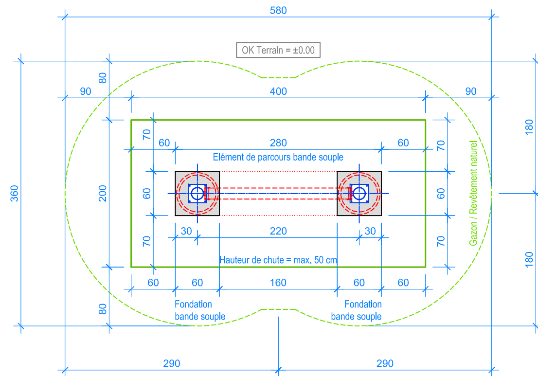
PLAN 1:50
