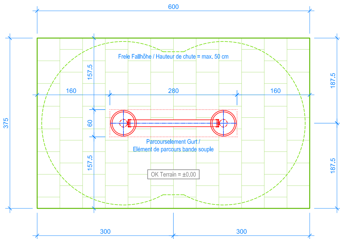
GRUNDRISS / PLAN 1:50
