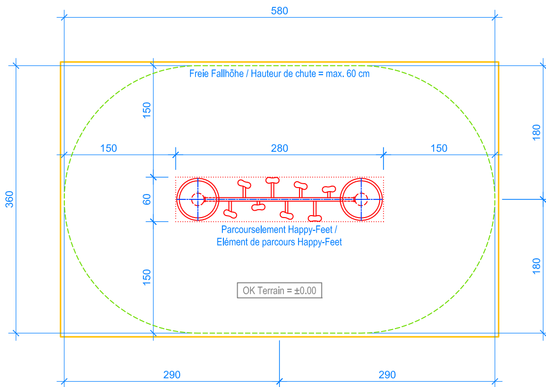
GRUNDRISS / PLAN 1:50
