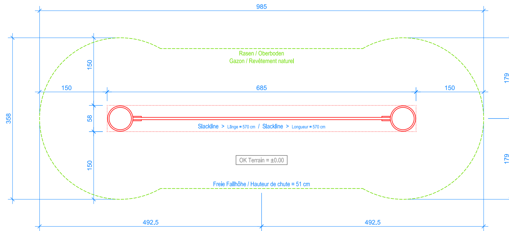
GRUNDRISS / PLAN 1:50
