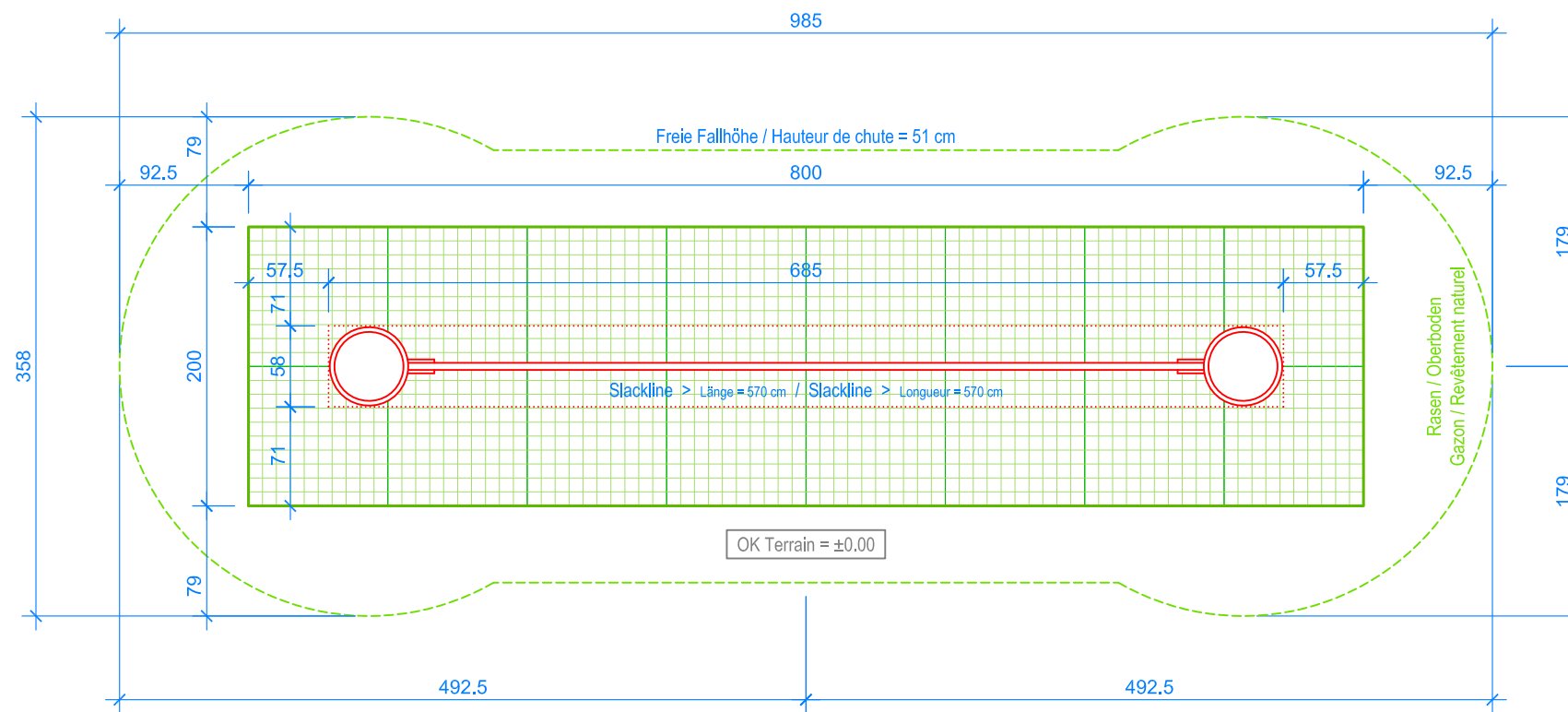
GRUNDRISS / PLAN 1:50
