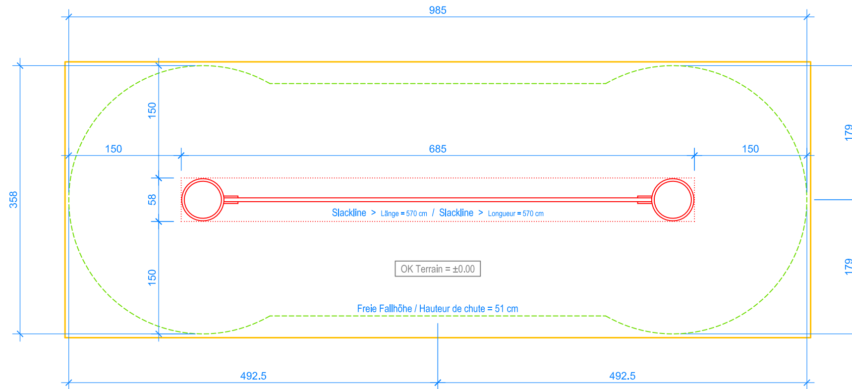
GRUNDRISS / PLAN 1:50
