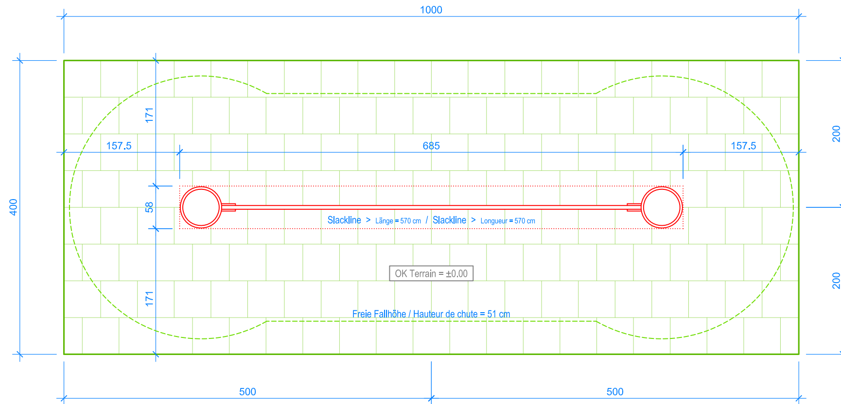
GRUNDRISS / PLAN 1:50
