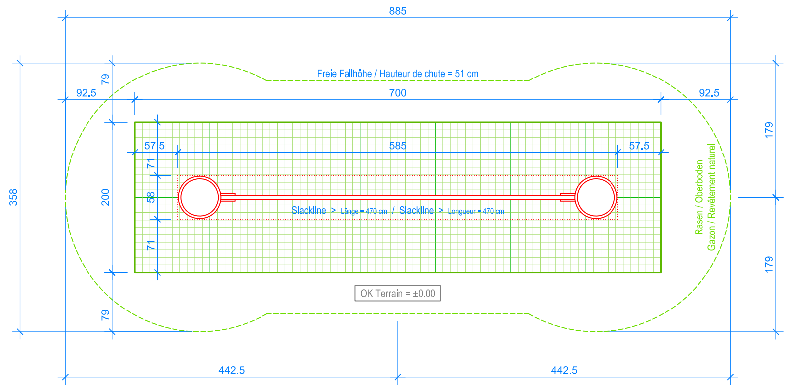
GRUNDRISS / PLAN 1:50
