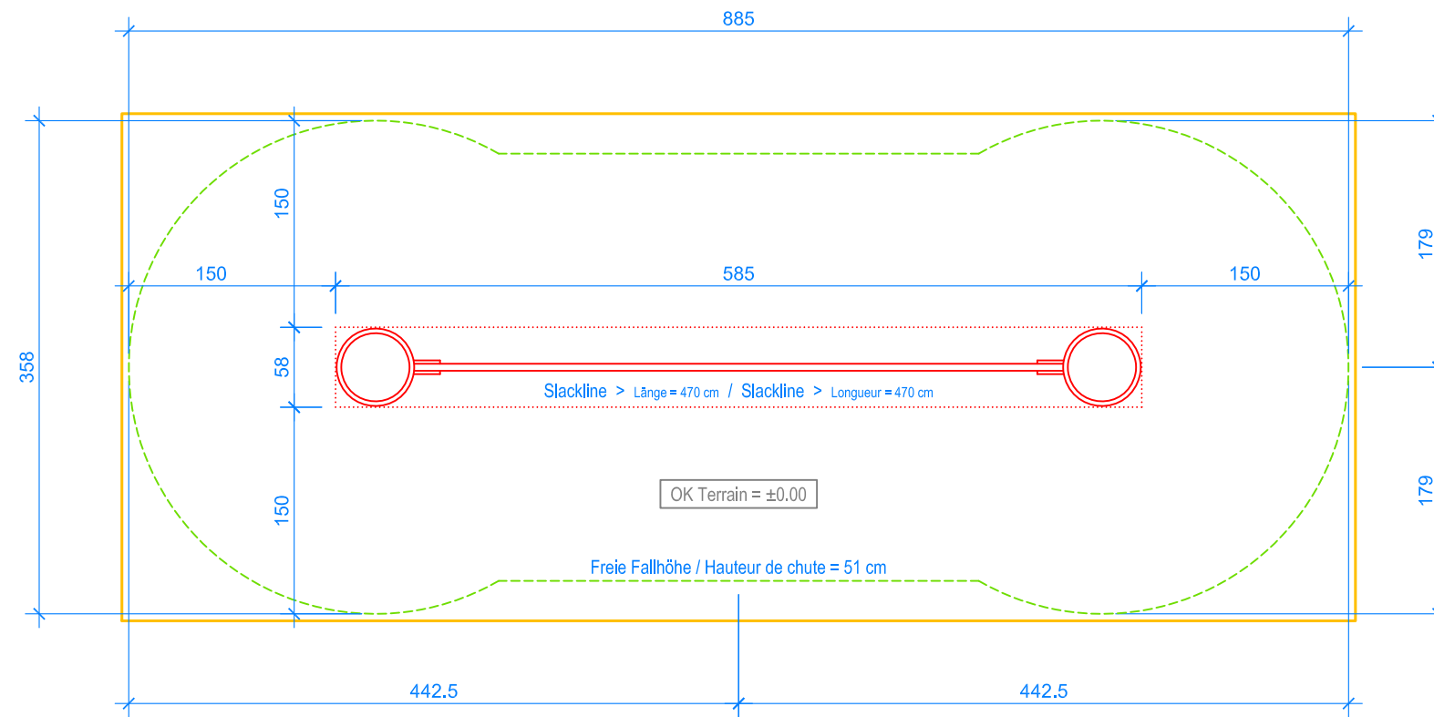
GRUNDRISS / PLAN 1:50
