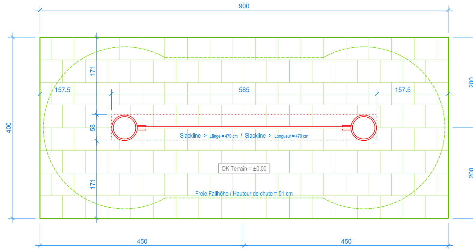
GRUNDRISS / PLAN 1:50
